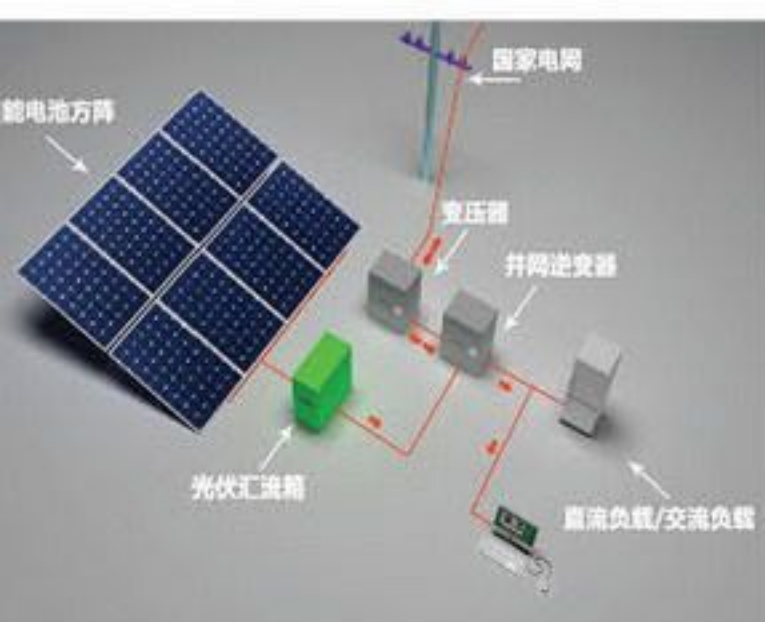
太阳能并网发电系统概要图
